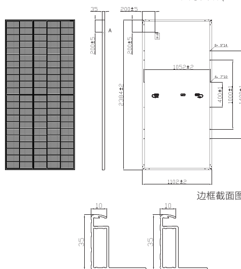
尺寸图纸 (mm)
